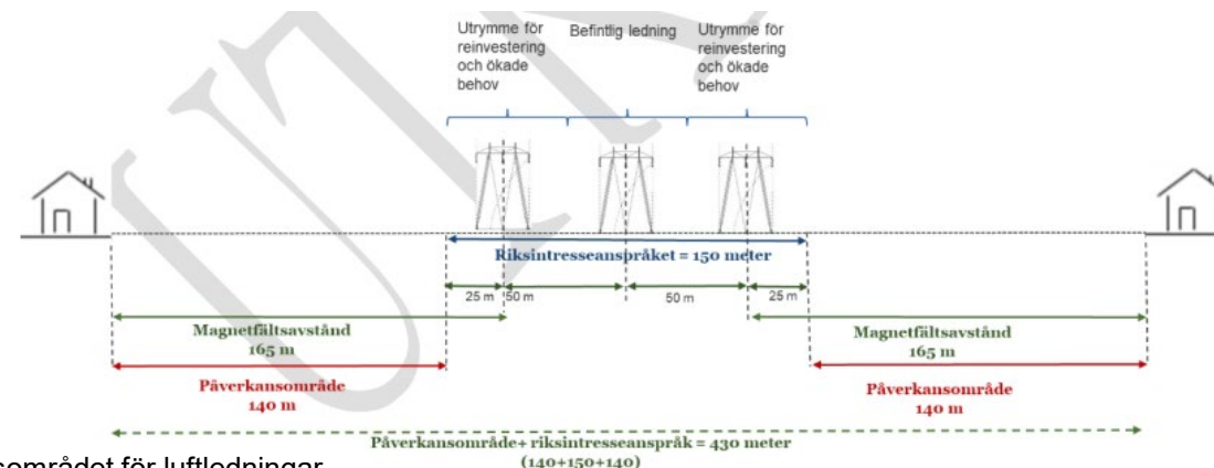
Föreslagna elledningar av riksintresse
